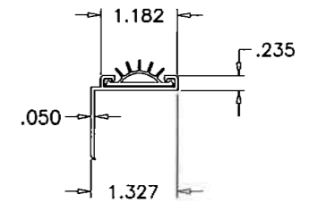
41 DOOR SWEEP (TOP)
